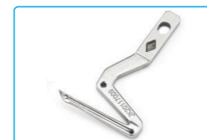
名 称: 下弯针 Description: Lower Looper 代 码/Part NO: 20117009 适 配: E3 5线 Machine Type: E3 series, 5thread model
