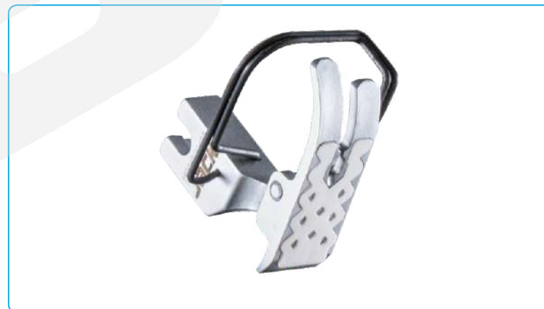
名称: 无影脚压脚 Description: Presser Foot 代 码/Part NO: 11601600100 适 配: A5E-B Machine Type: A5E-B
