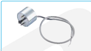
名称: 剪线电磁铁组件 Description: Wire Cutting Solenoid 代码/Part NO: 11463000600 适配: A5E-A/A5E-B Machine Type: A5E-A/A5E-B
