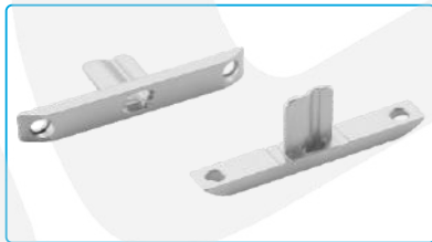
名称: 双针针板片(1.2-1.8) Description: Needle Hole Plate (1.2-1.8) 代码/Part NO: 155315016 适配: 全系双针(短线头除外) Machine Type: Post-bed Double Needle Machine (Except-X)
