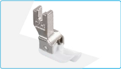
名称: TCR压脚组件 1/16E Description: TCR Presser Foot 1/16E 代码/Part NO: 813777 适配: 平缝机通用 Machine Type: All lockstitch machine series
