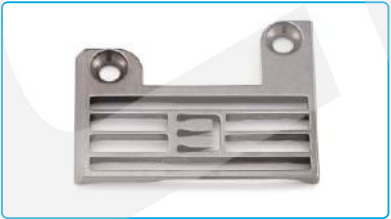
名称: 针板(01CB) (364) Description: Needle Plate (01CB, 364) 代码/Part NO: 30715006 适配: 8670系列-01CB机型 Machine Type: 01CB type for 8670 series
