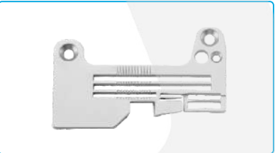
名称: 四线针板 (2×6) Description: NEEDLE PLATE 代码/Part NO: 121115011 适配: C5-4 Machine Type: C5-4
