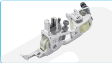
名称: JK-A10带轮压脚 (小号) Description: Presser Foot JK-A10(S) 代 码/Part NO: 800016 适 配: 平缝系列 Machine Type: Lockstitch Series
