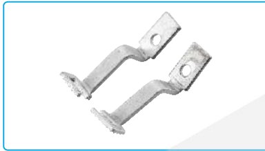
名称: 厚料压脚组件 (25*5) Description: Presser Foot Assy.(25*5) 代 码/Part NO: 40316015+40316016 适 配: JK-T1900BH Machine Type: JK-T1900BH
