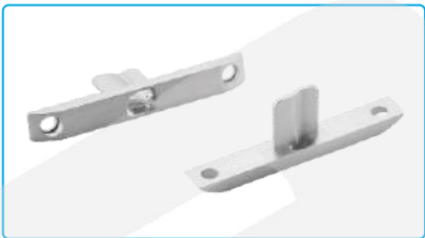
名称: 双针针板片(2.0-2.4) Description: Needle Hole Plate (2.0-2.4) 代码/Part NO: 155315007 适配: 全系双针(短线头除外) Machine Type: Post-bed Double Needle Machine (Except-X)
