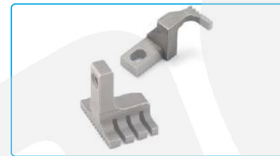
名称: 牙齿组件 Description: Feed Dog Assy 代 码/Part NO: 30214008 + 30214009 适 配: W4/W4S/K4/K5系列-02BB机型 Machine Type: 02BB type for W4/W4S/K4/K5 series
