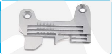
名称: 针板(倒回缝) Description: Needle Plate (BK) 代码/Part NO: 20715019 适配: E4/E4S-3-82/233 Machine Type: E4/E4S-3-82/233
