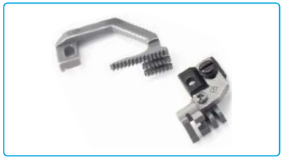
名称: 牙齿组件 Description: Feed Dog Assy 代 码/Part NO: 2011401900 适 配: E3-5-M2-35 Machine Type: E3-5-M2-35
