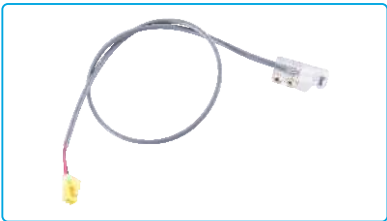
名称: 第三接收 Description: Sensor 代 码/Part NO: 21130303 适 配: C5-BK/C5T Machine Type: C5-BK/C5T
