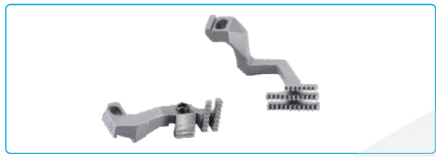
名称: 四线牙齿组件 Description: FEED DOG ASM. 代 码/Part NO: 2041400600 适 配: JK-797三四线系列 Machine Type: JK-797-3/4
