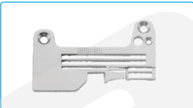
名称: 四线针板 (2×5) Description: NEEDLE PLATE 代码/Part NO: 121115009 适配: C5-4 Machine Type: C5-4
