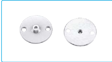
名称: 小针板(Φ1.8,T2.0) Description: NEEDLE HOLE PLATE(Φ1.8,T2.0) 代 码/Part NO: 41815011 适 配: 模板机系列 Machine Type: Template Machine Series
