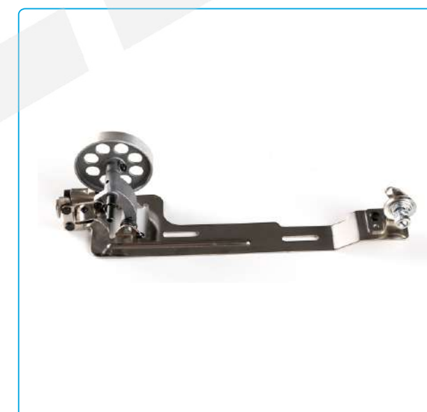
名称: 绕线器组件 Description: Bobbin Winder 代码/Part NO: 1013100600 适配: JK-8720 Machine Type: JK-8720
