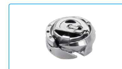
名称: 旋梭组件 Description: Hook Asm. 代码/Part NO: 15581800300 适配: S7-92-T Machine Type: S7-92-T
