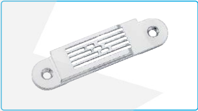
名称: 三针针板 (1/8, 五排齿) Description: Needle Plate(1/8) 代 码/Part NO: 112615002 适 配: JK-8560G Machine Type: JK-8560G
