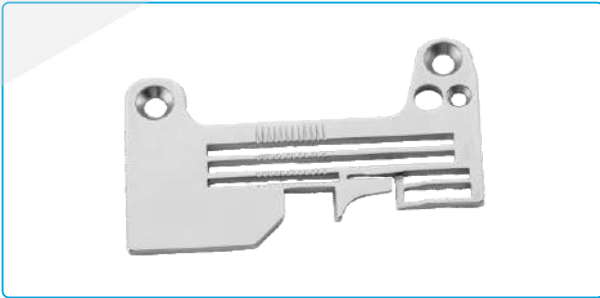
名称: 针板(倒回缝) Description: Needle Plate (BK) 代码/Part NO: 20715019 适配: E4/E4S-3-82/233 Machine Type: E4/E4S-3-82/233
