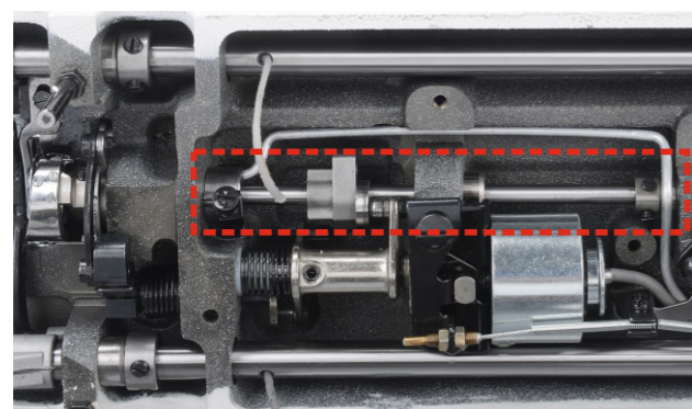
1 Alzapiedino Automatico, più efficienza Rasafilo automatico, diminuisce i costi automenta l'efficienza del lavoro
